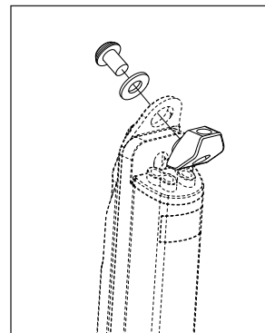
Adattatore per installazione rovesciata PU EPS V2
