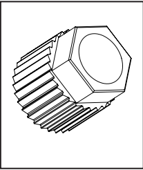
T-22 Attrezzo per smontaggio cremagliera - Road Hub rachet ring tool - Road Outil pour le demontage de la cremaillere - Road
