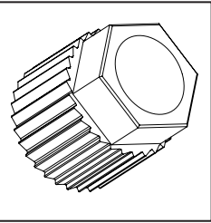
T-23 Attrezzo per smontaggio cremagliera - Mtb Hub rachet ring tool - Mtb Outil pour le demontage de la cremaillere - Mtb
